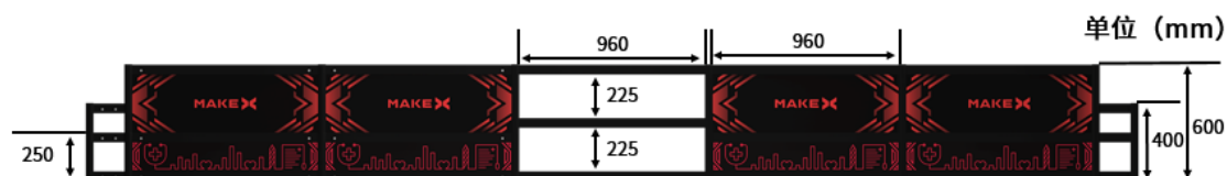
图 3.3-5 中央隔栏尺寸图
