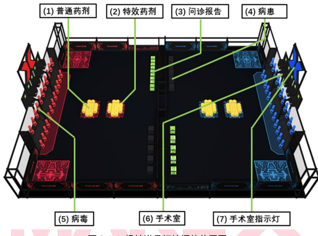
图 3.4-1 场地道具初始摆放位置图
