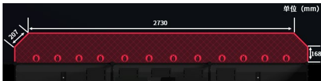
图 3.3-3 病毒隔离区俯视尺寸图
